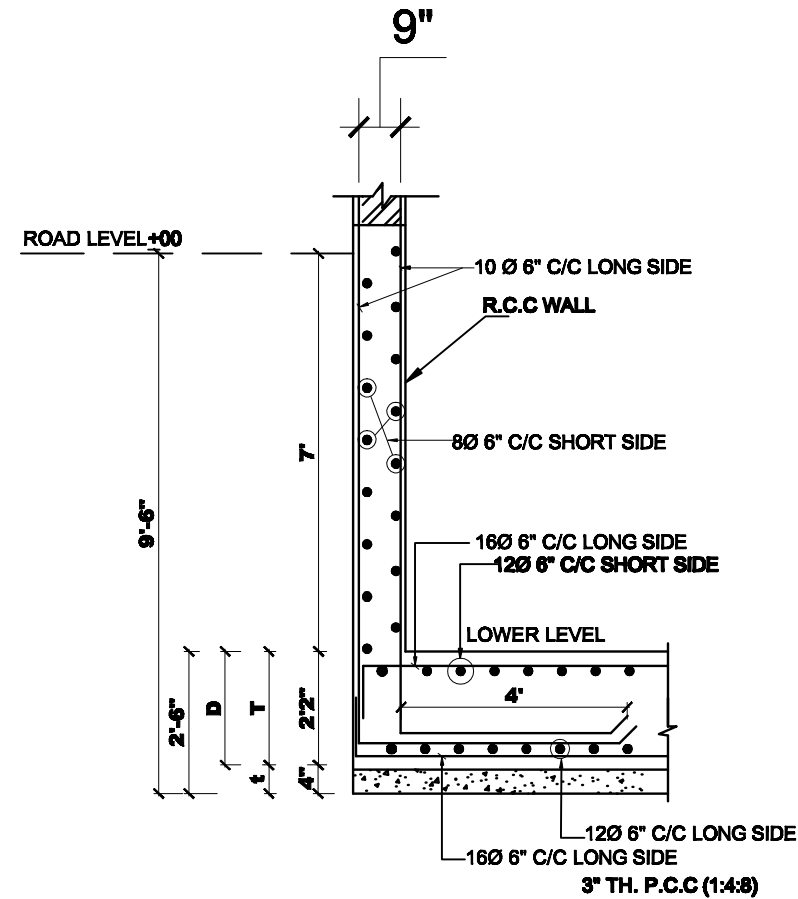
RCC HEIGHT DET.
